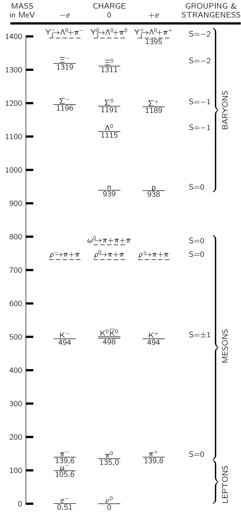
图 2.1: 基本粒子
